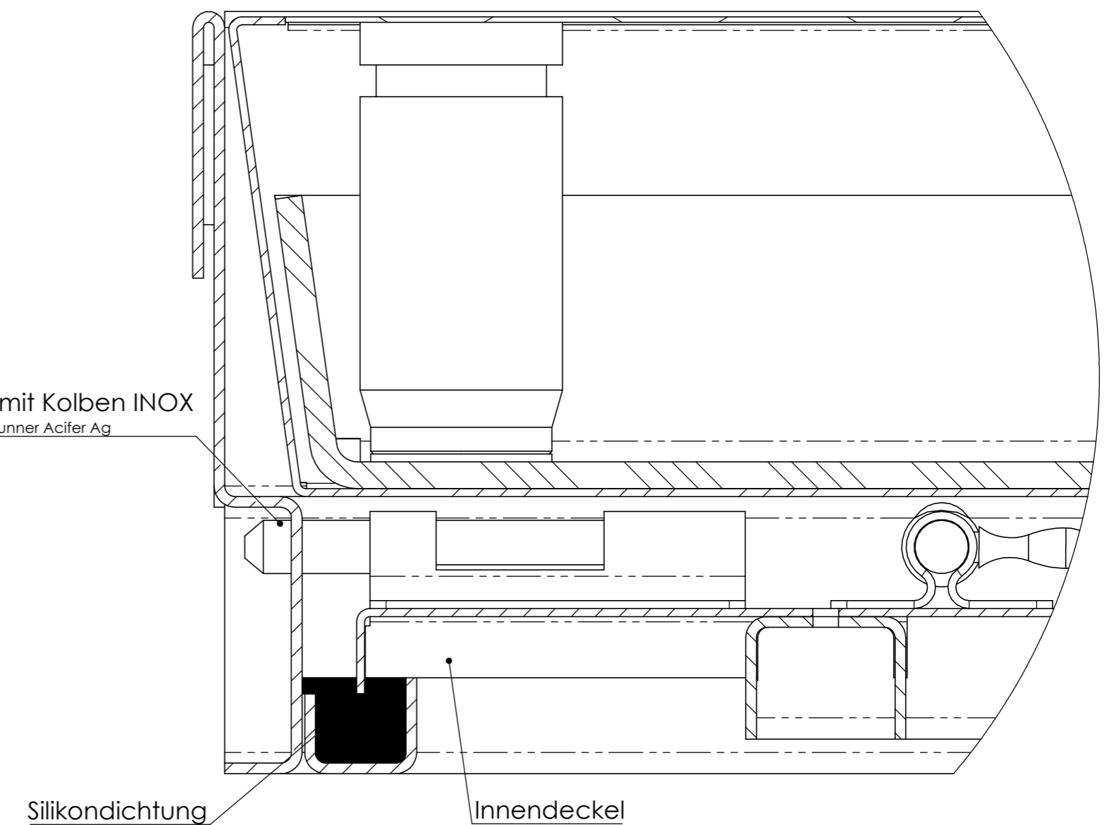
DETAIL C MABSTAB 1 : 1
